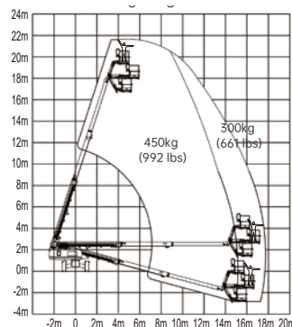
Pracovní rozsah T20J-H
