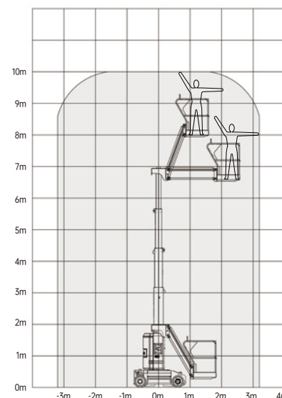
Pracovní dosahy M0810JE
