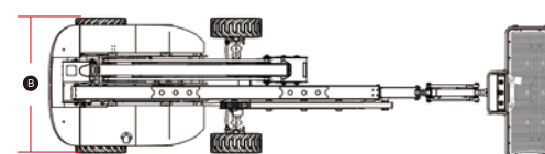
Pracovní rozsah AR20J
