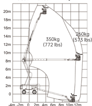
Pracovní rozsah AR20J
