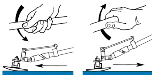
Ovládání úhlu lišty obslužnou tyčí
